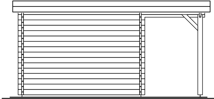
zijaanzicht (l) / side view (l)
