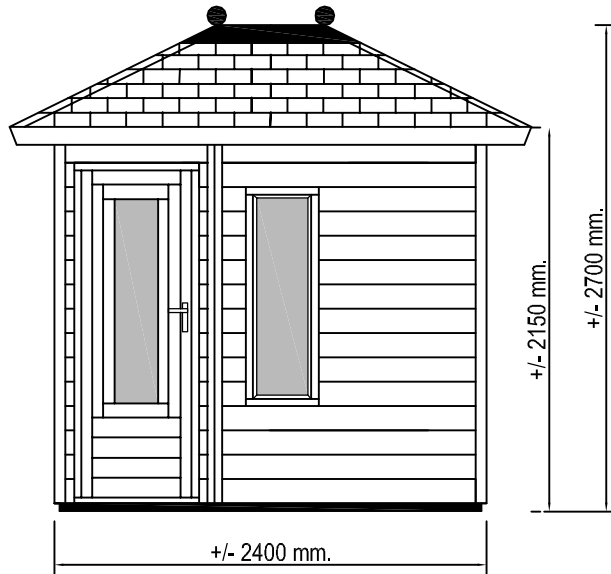
Voor aanzicht Vorder ansicht Front view
