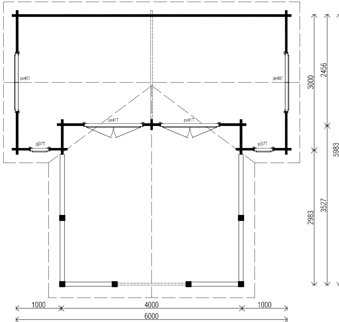
plattegrond / plan
